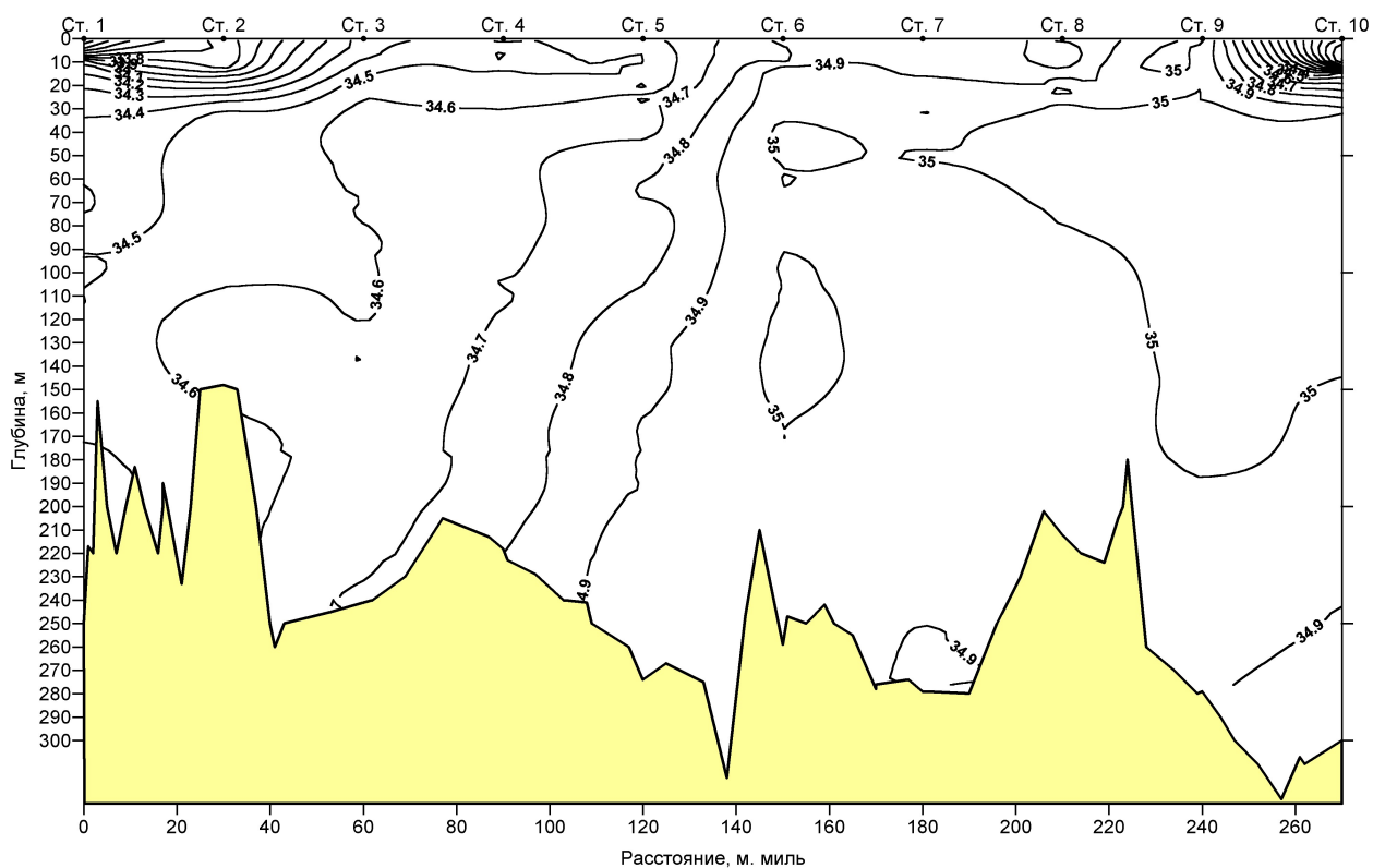
Рис. 4. Распределение солености воды (‰) на ст. 1-10 разреза "Кольский меридиан" (7-9 августа 2003 г.)
