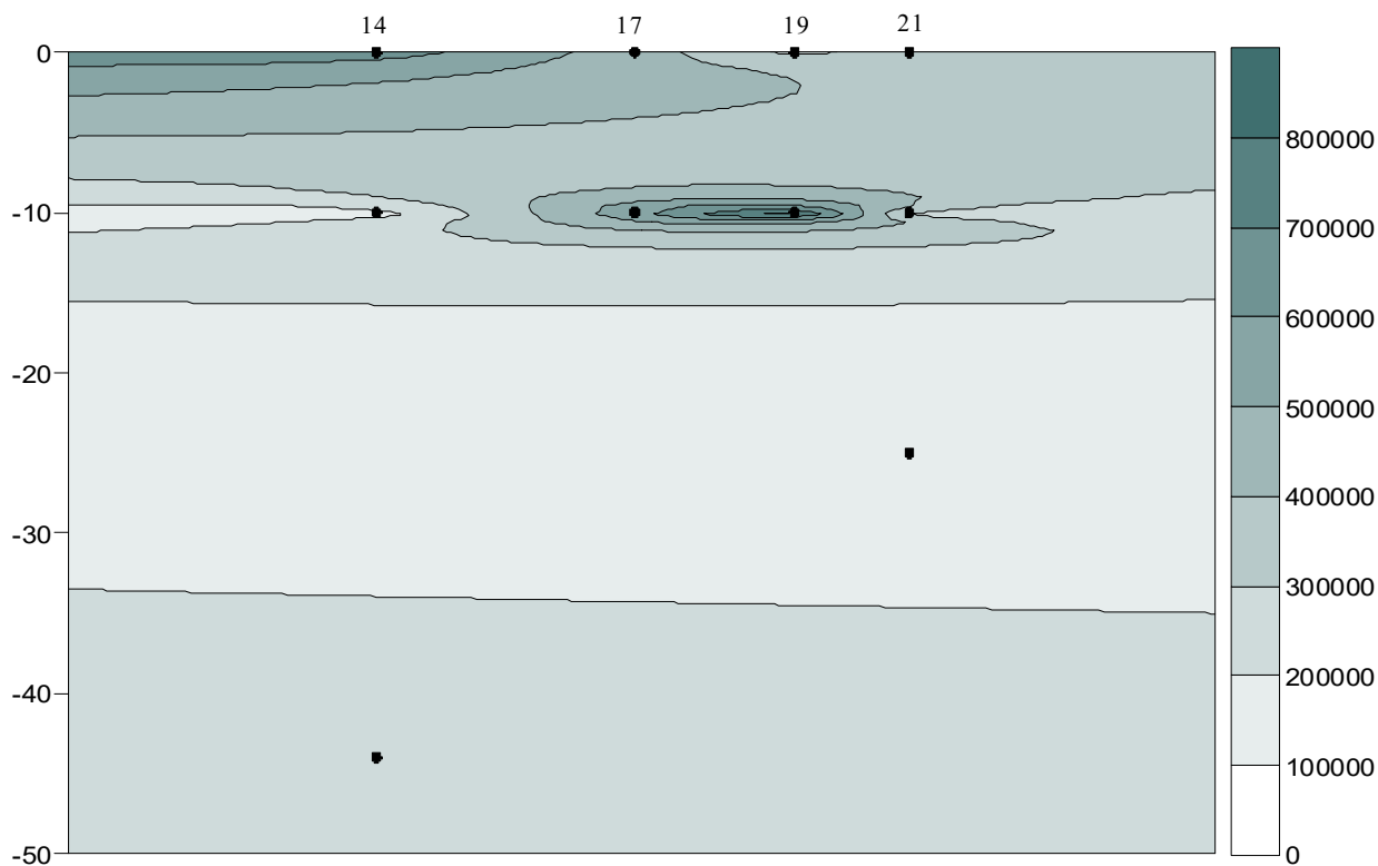
Рис. 16 Пространственное распределение численности нанопланктона в верхнем 50-метровом слое на разрезе Норд - Кап – о-в Медвежий (ст. 14-21).
