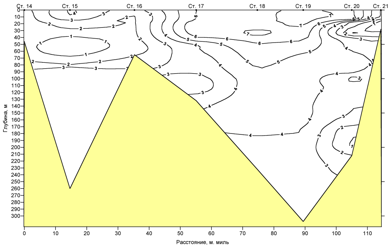
Рис. 7. Распределение температуры ( ^{\circ}\text{C} ) воды на ст. 14-21, XIX разрезе (10 - 11 августа 2003 г.)
