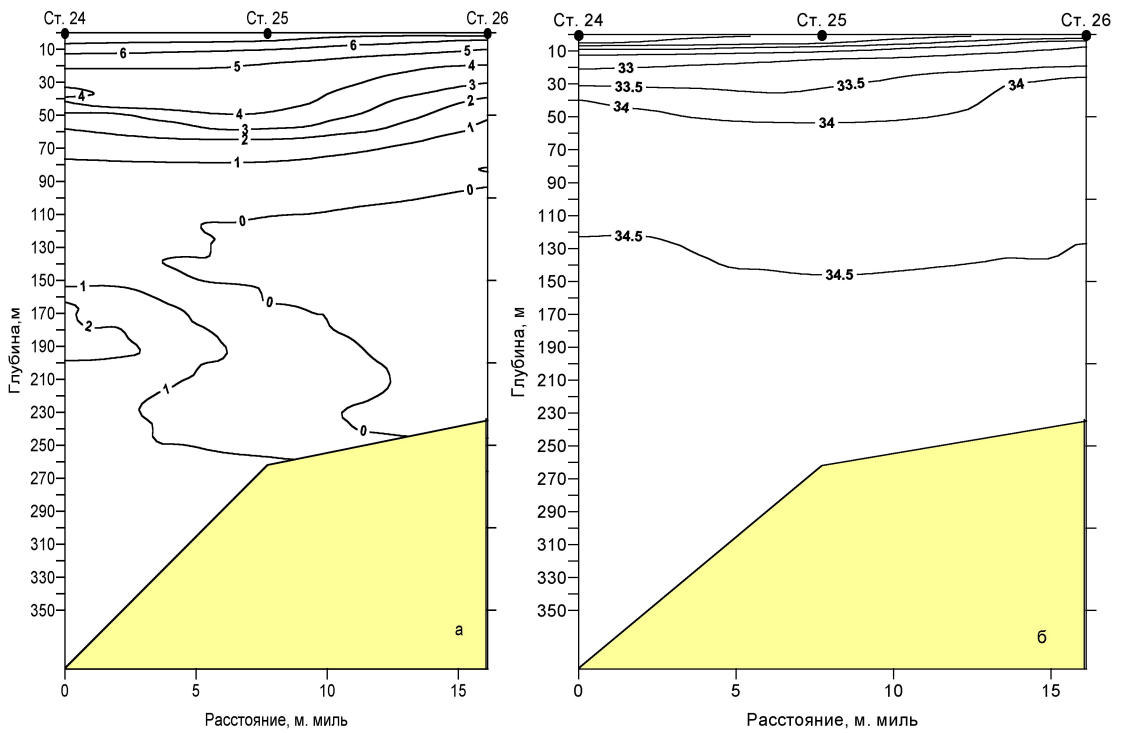
Рис. 9. Распределение температуры ( ^{\circ}\text{C} , а) и солёности ( \text{‰} , б) воды на ст. 24-26, разрезе в Ис-фьорде (12 августа 2003 г.)
