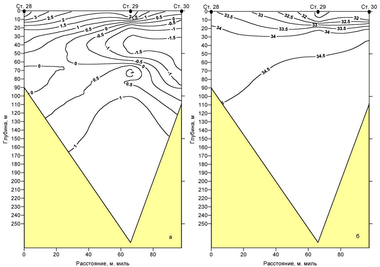
Рис. 10. Распределение температуры ( ^{\circ}\text{C} , а) и солёности ( \text{‰} , б) воды на ст. 28-30 XXVIII разрезе (14 августа 2003 г.)
