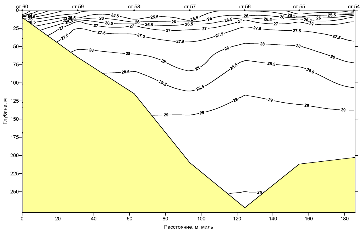
Рис. 15. Распределение солености воды (‰) на разрезе по ст. 54-60 (23-24 августа 2003 г.)
