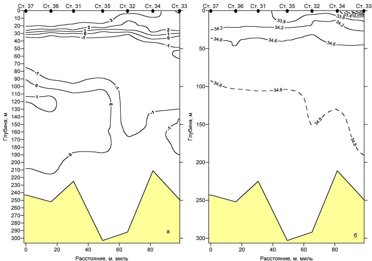
Рис. 11. Распределение температуры ( ^{\circ}\text{C} , а) и солёности ( \text{‰} , б) воды на разрезе по ст. 37, 36, 31, 35, 32, 34 и 33 в северно-восточной части Баренцева моря (16 - 17 августа 2003 г.)
