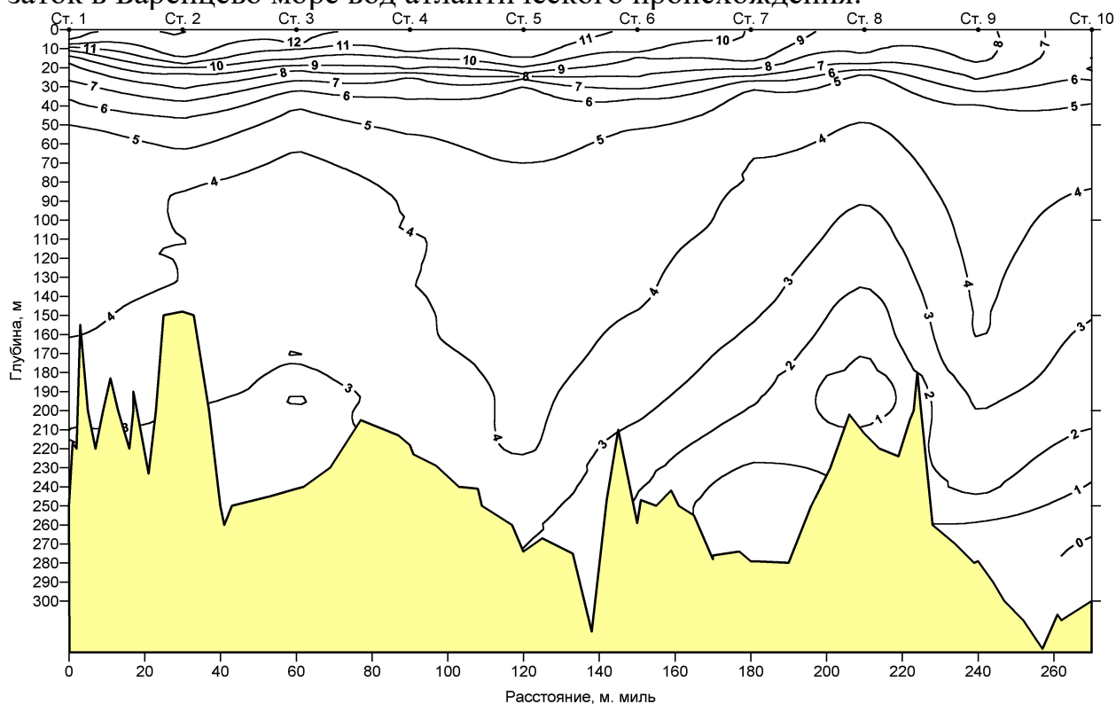
Рис. 3. Распределение температуры воды (°C) на ст. 1-10 разреза "Кольский меридиан" (7-9 августа 2003 г.)
