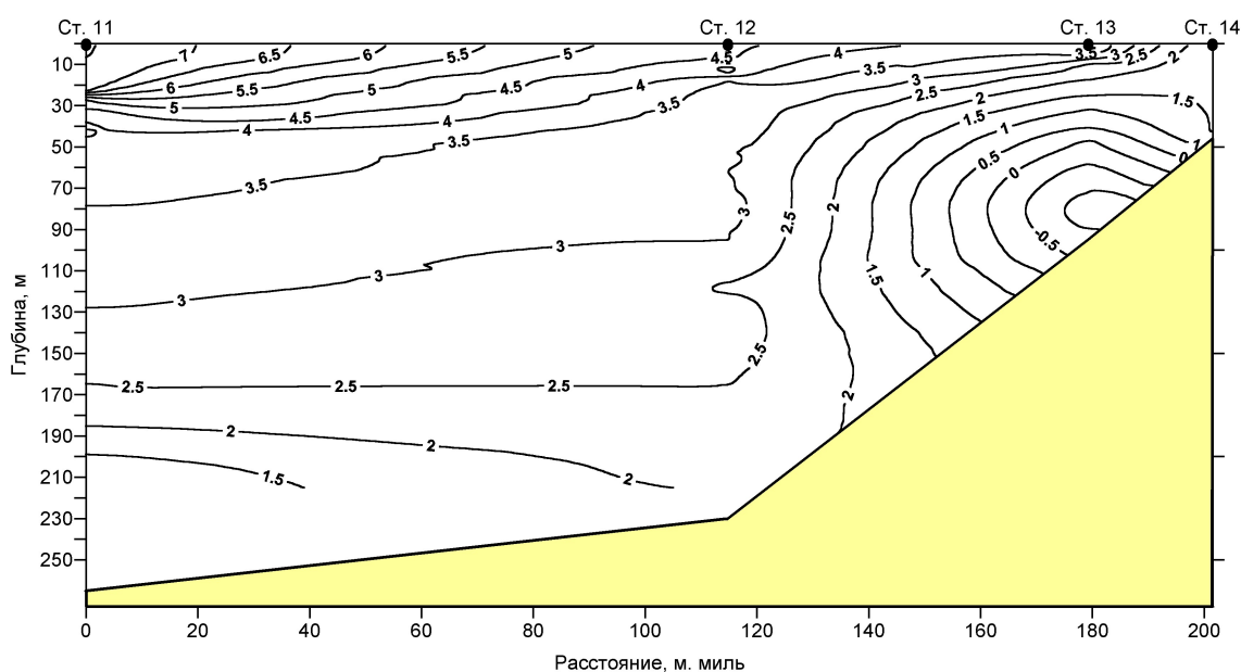
Рис. 5. Распределение температуры воды (°C) на ст. 11-14 XXIX и XIX разрезов (9 - 10 августа 2003 г.)
