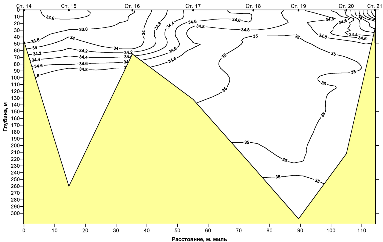
Рис. 8. Распределение солёности (‰) воды на ст. 14-21, XIX разрезе (10 - 11 августа 2003 г.)
