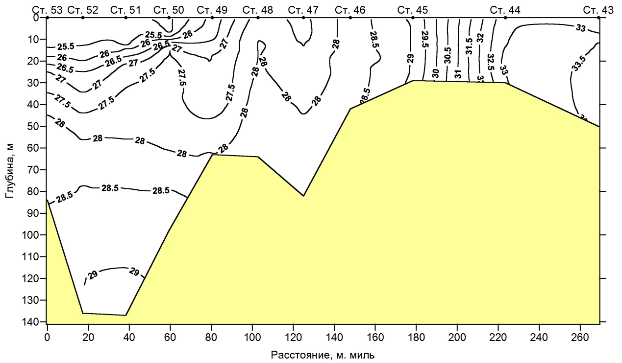
Рис. 13. Распределение солености воды (‰) на разрезе по ст. 43-53 (20-22 августа 2003 г.)
