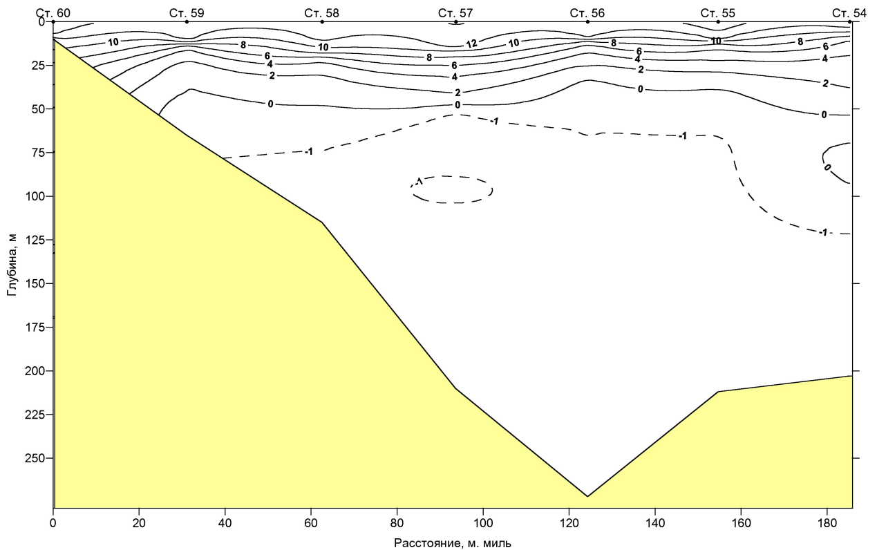
Рис. 14. Распределение температуры воды (°C) на разрезе по ст. 54-60 (23-24 августа 2003 г.)
