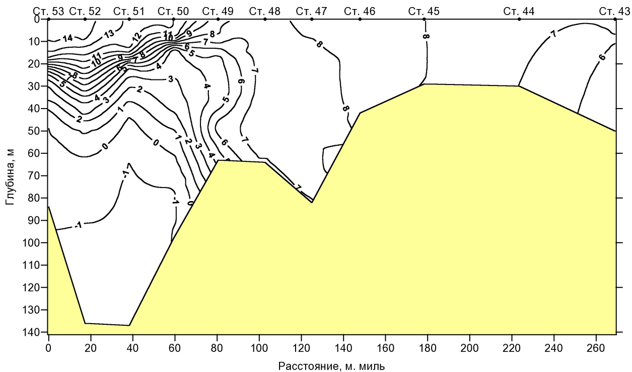
Рис. 12. Распределение температуры воды ( ^{\circ}\text{C} ) на разрезе по ст. 43-53 (20-22 августа 2003 г.)
