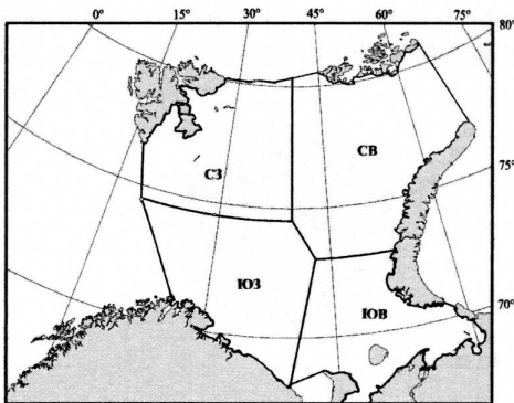
Рис. 2. Однородные ледовые районы Баренцева моря (Жичкин, 2012)
