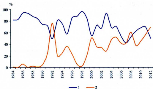
Рис. 6 Динамика ледовитости (%) в марте-апреле (1) и промышленного значения (%) высокоширотных районов Баренцева моря в августе-ноябре (2)
