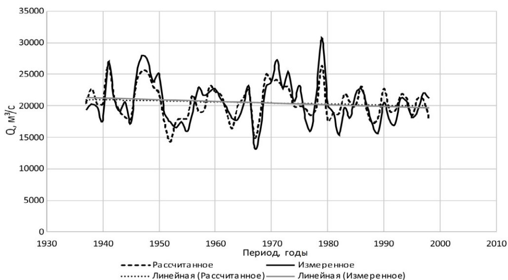
Рис. 1. Средние расходы воды в створе гидрологического поста “Салехард” в теплое полугодие по данным натурных измерений и рассчитанные на основе множественной регрессии
