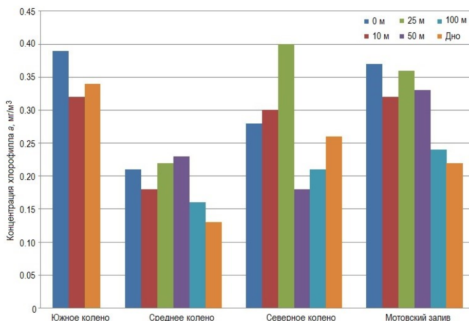
Рис. 3. Средняя концентрация хлорофилла a в слоях водной толщи в Кольском и Мотовском заливах в октябре 2017 г. (Водопьянова, Духно, 2018)
