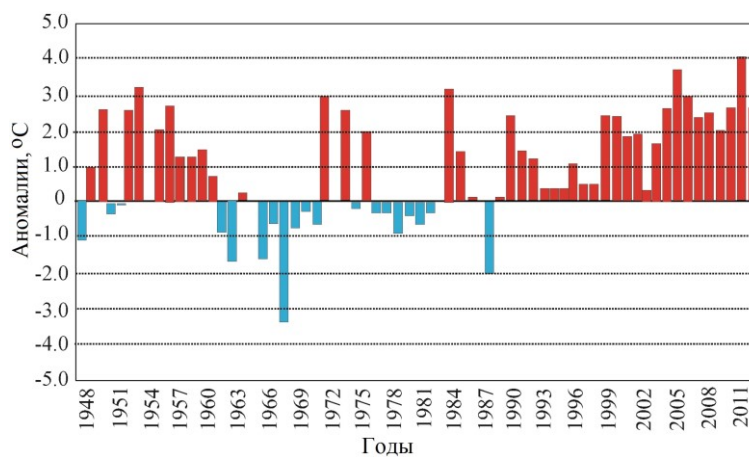
Рис. 2. Аномалии среднегодовой температуры воздуха (январь–декабрь 1948–2013 гг.) по данным ЗГМО “Баренцбург” (Анциферова и др., 2014)
